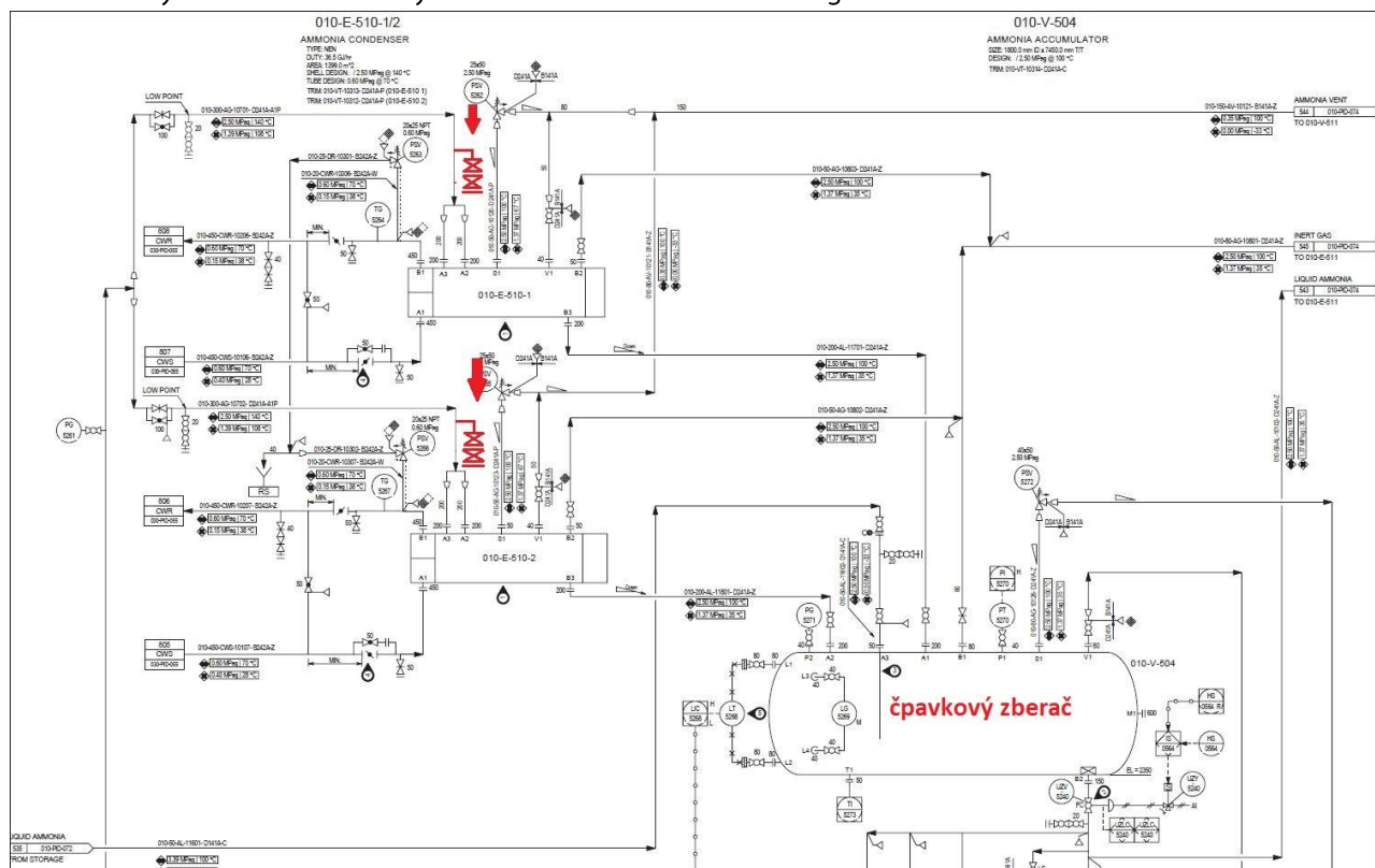
Obr. č. 1 – vyznačenie navrhovaných odvzdušňovacích ventilov na tg. schéme
