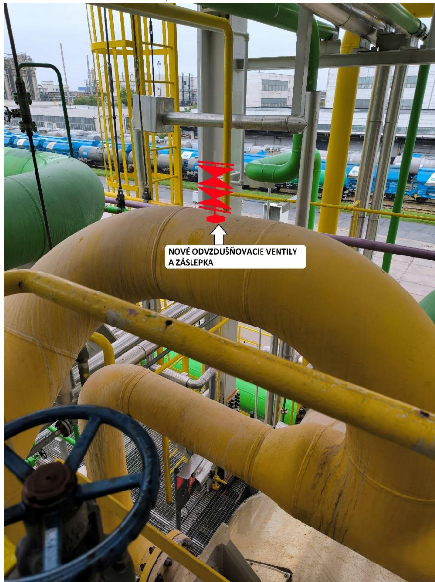
Obr. č. 3 - návrh inštalácie na potrubí 010-300-AG-10702 smerom do E-510-2
